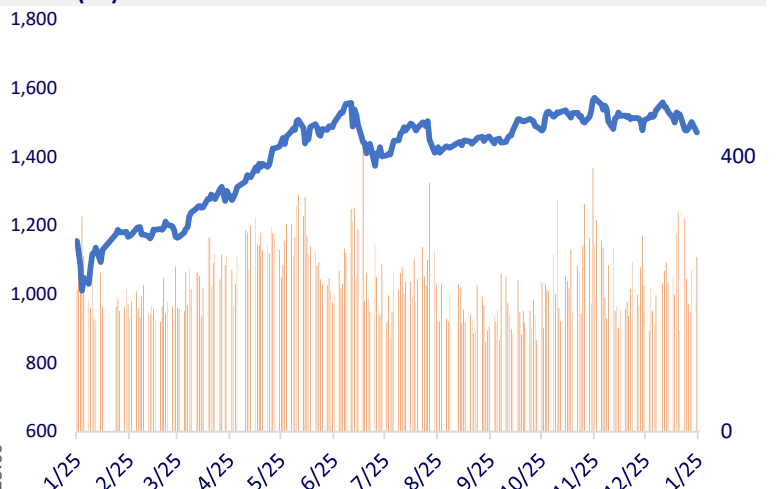
VN30 (1Y)
