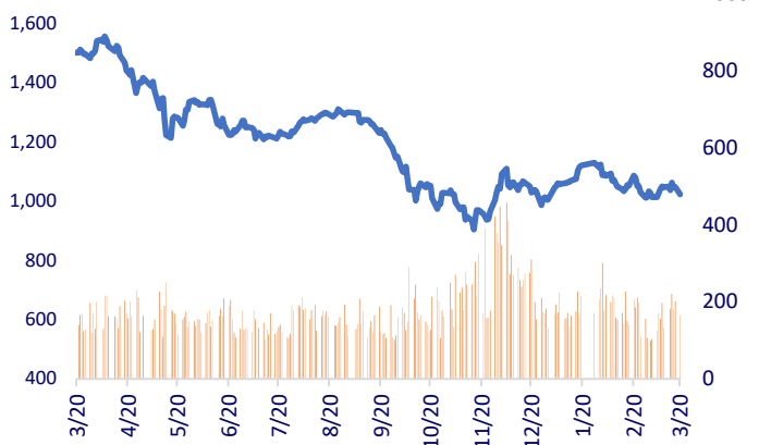
VN30 (1Y)
