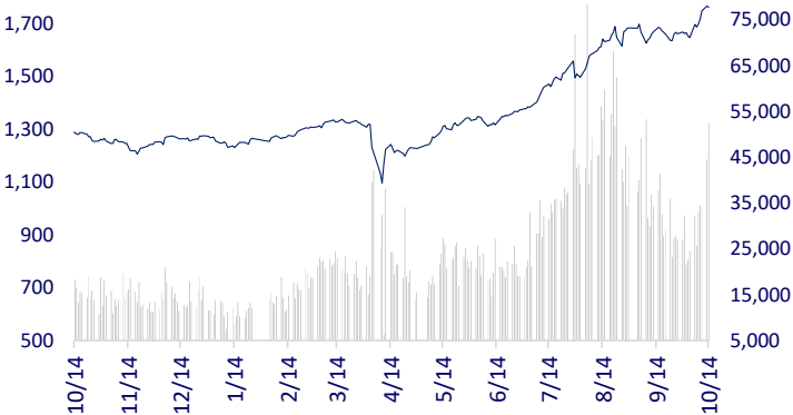
VNINDEX (1Y)
