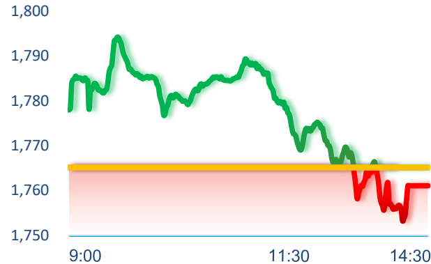
VNINDEX - INTRADAY
